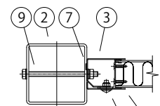
C-C 断面図 (1/8)
