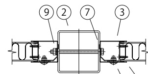
D-D 断面図 (1/8)
