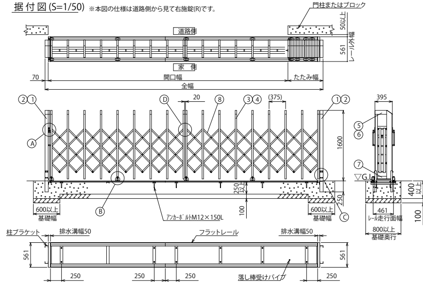
据付図 (S=1/50) ※本図の仕様は道路側から見て右旋錠(R)です。
