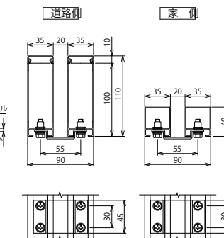
(D) 枠体連結部詳細図(S=1/5)
