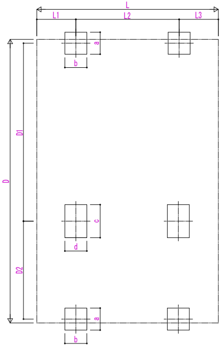
■基礎配置図
