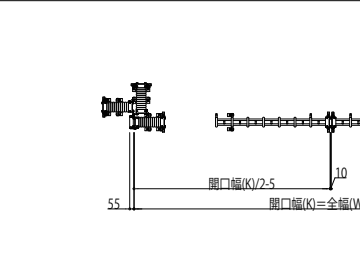
レイオス5型片開き 平面図
