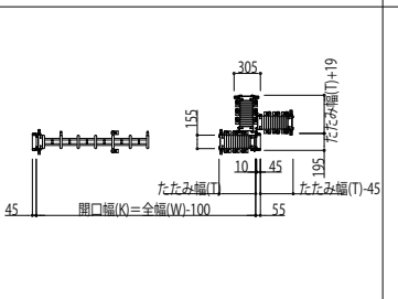
レイオス7型両開き 平面図
