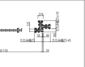
レイオス5型両開き 平面図
