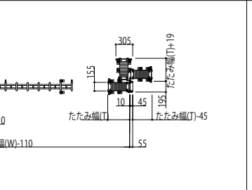
レイオス7型片開き 平面図
