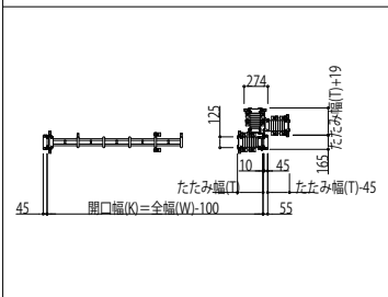
レイオス5型片開き 平面図
