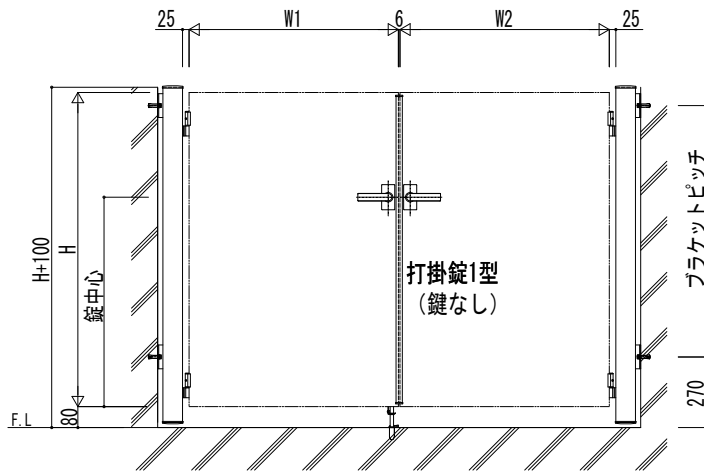
調整用スペーサー無しの場合シングル落とし錠仕様
