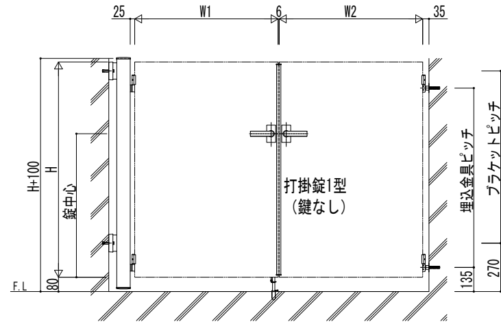
調整用スペーサー有りの場合 シングル落とし錠仕様
