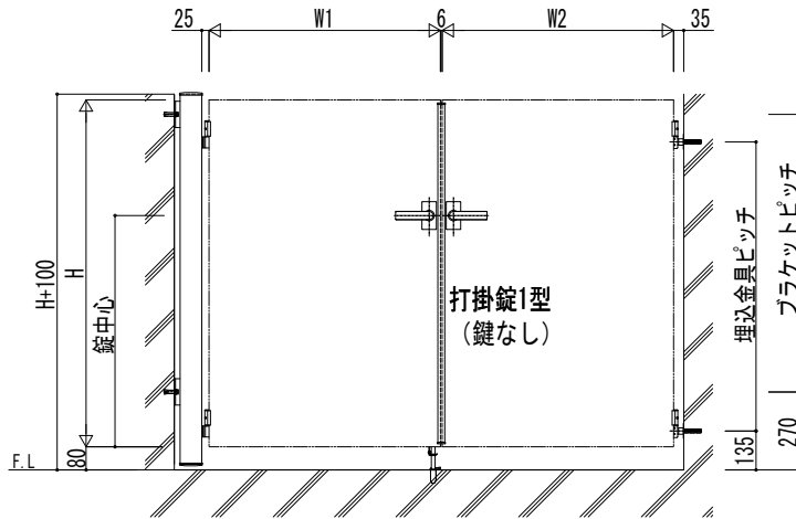
調整用スペーサー無しの場合 シングル落とし錠仕様
