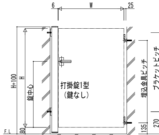
調整用スペーサー無しの場合
