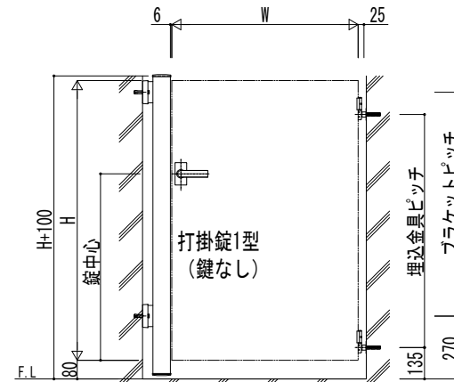
調整用スペーサー有りの場合
