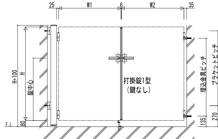
調整用スペーサー有りの場合 シングル落し錠仕様
