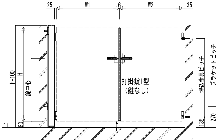
調整用スペーサー無しの場合 シングル落し錠仕様
