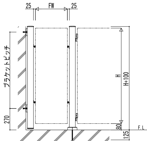
□120 内開き 調整用スペーサー無しの場合
