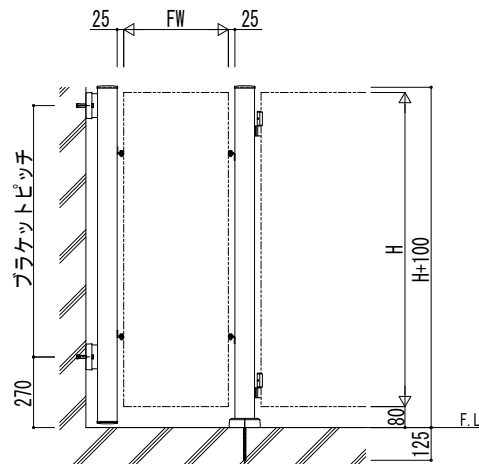
□120 内開き 調整用スペーサー有りの場合
