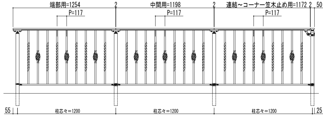
端部用本体
