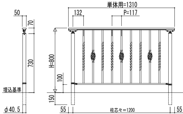
単体用本体
