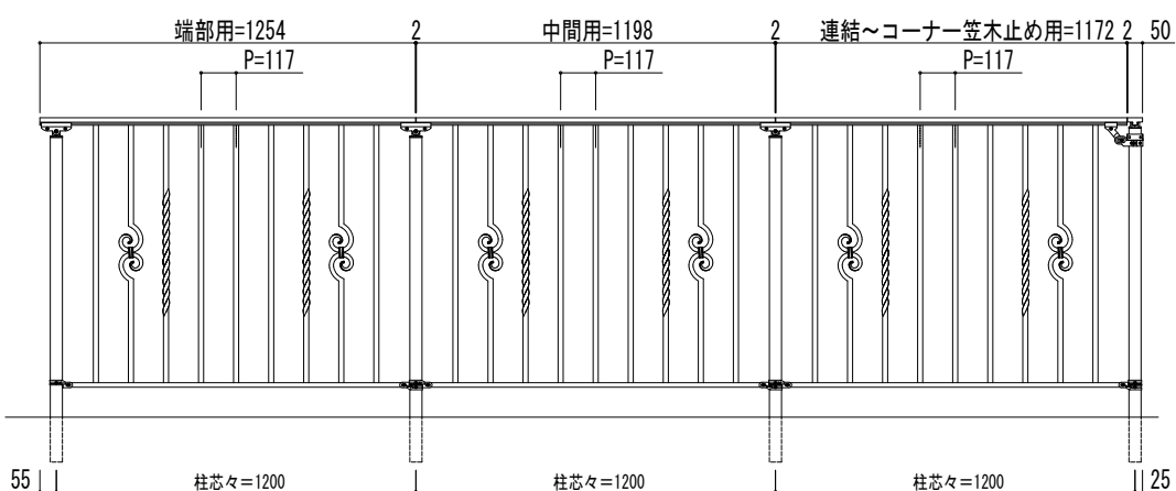
端部用本体
