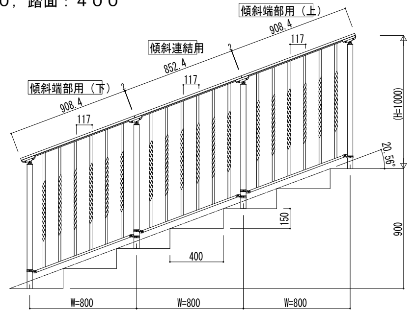
③ 蹴上げ：150，踏面：400
