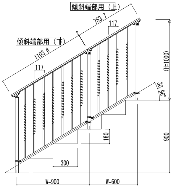
② 蹴上げ：180，踏面：300
