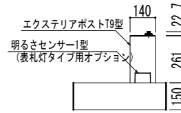
エクステリアポストT9型（前入れ・後ろ出し）組合せの場合
