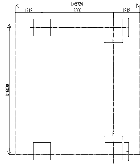
■ 基礎寸法表
