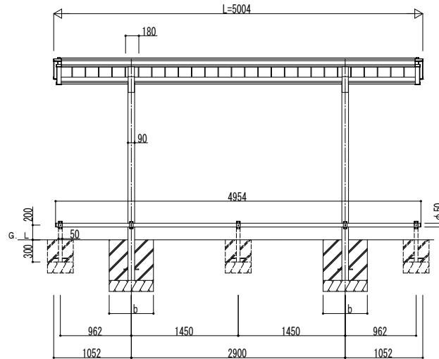
■ 基礎寸法表
