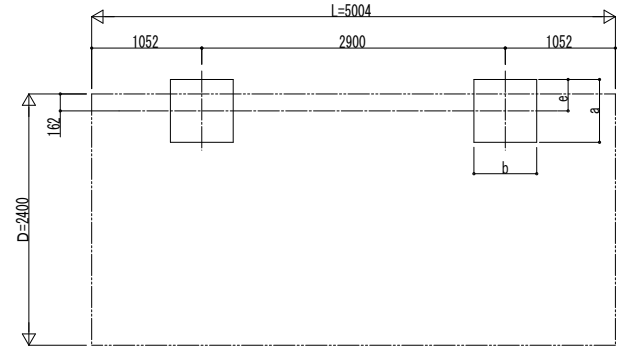
■ 基礎配置図
