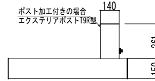
エクステリアポストT9R型（前入れ・横出し）組合せの場合
