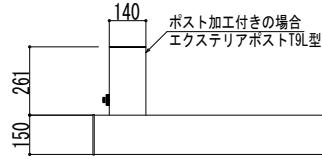
エクステリアポストT9L型（前入れ・横出し）組合せの場合
