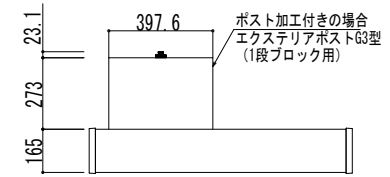
エクステリアポストG3型 (1段ブロック用) 組合せの場合
