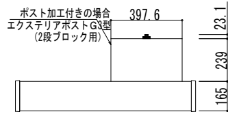
エクステリアポストG3型 (2段ブロック用) 組合せの場合
