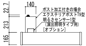
エクステリアポストT9型 (前入れ・後ろ出し) 組合せの場合
