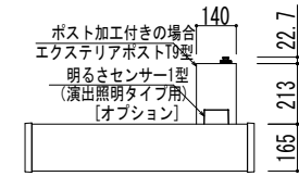
エクステリアポストT9型 (前入れ・後ろ出し) 組合せの場合
