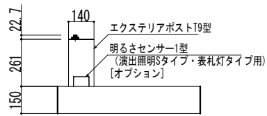
エクステリアポストT9型（前入れ・後ろ出し）組合せの場合
