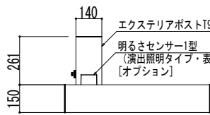
エクステリアポストT9L型（前入れ・横出し）組合せの場合
