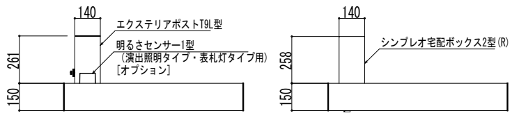
エクステリアポストT9L型（前入れ・横出し）組合せの場合
