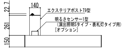
エクステリアポストT9型（前入れ・後ろ出し）組合せの場合
