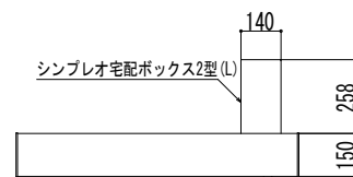
シンプル宅配ボックス2型 (L) 組合せの場合
