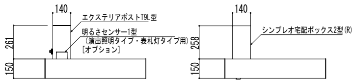
エクステリアポストT9L型（前入れ・横出し）組合せの場合 シンプレオ宅配ボックス2型(R)組合せの場合
