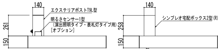
エクステリアポストT9L型（前入れ・横出し）組合せの場合 シンプル宅配ボックス2型(R)組合せの場合
