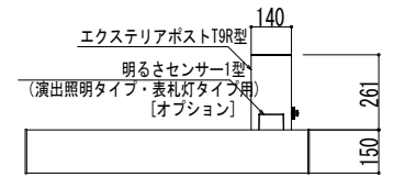
エクステリアポストT9R型（前入れ・横出し）組合せの場合
