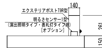
エクステリアポストT9R型（前入れ・横出し）組合せの場合
