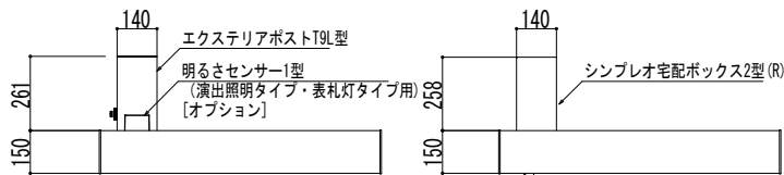
エクステリアポストT9L型（前入れ・横出し）組合せの場合 シンプルオ宅配ボックス2型 (R) 組合せの場合
