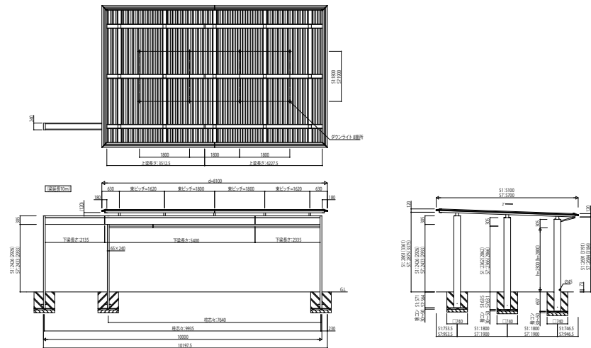
3台用 積雪30cm仕様 梁延長タイプ
