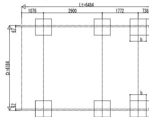
■ 基礎配置図
