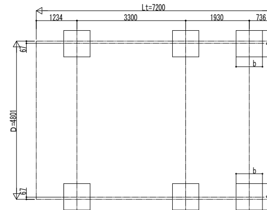
■ 基礎配置図
