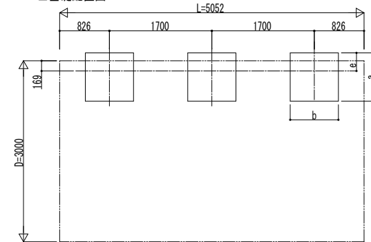
■ 基礎配置図
