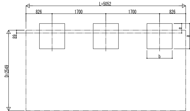
■基礎配置図
