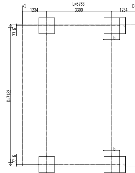
■ 基礎配置図
