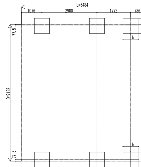
■ 基礎配置図
