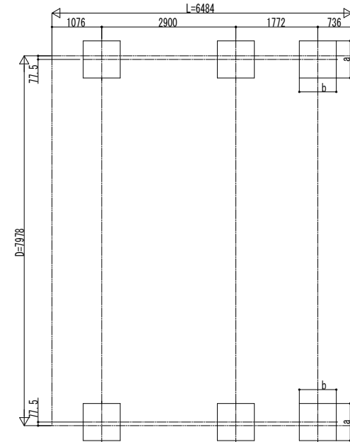
■基礎配置図
