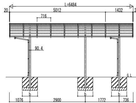
■基礎寸法表
