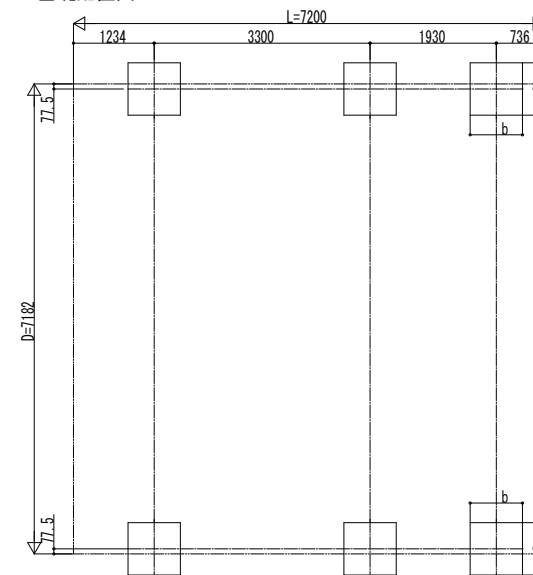
■ 基礎配置図
