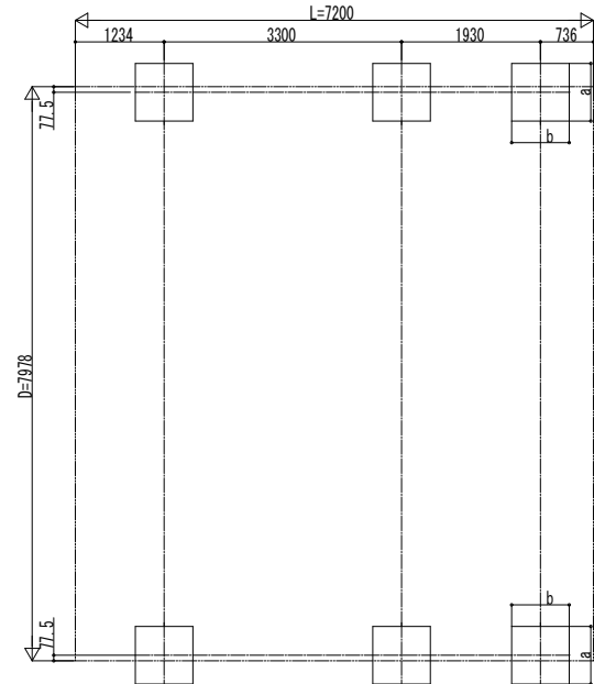
■基礎配置図
