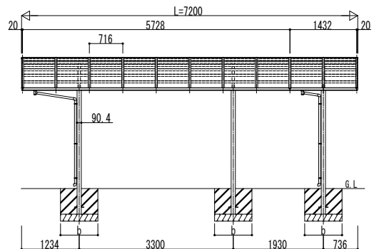
■基礎寸法表
