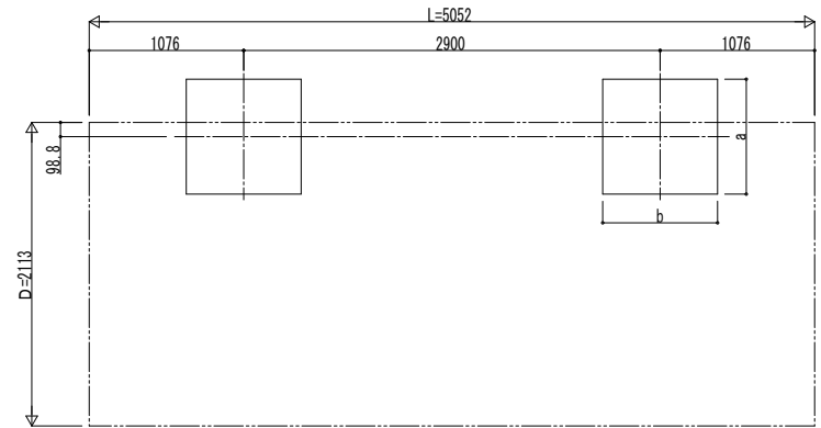
■ 基礎配置図
