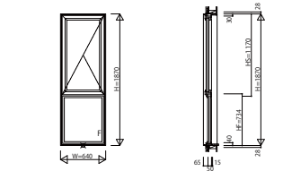
たてすべり出し窓部
