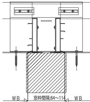
単窓および段窓ランマ通し雨戸の場合
