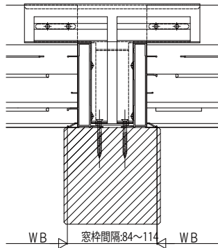
段窓無目下部雨戸の場合
