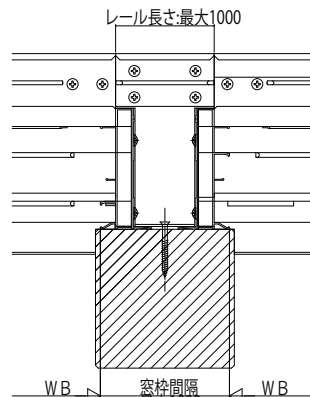
WB 窓枠間隔:最大1022 WB
