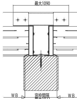
段窓無目下部雨戸の場合
