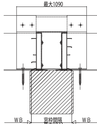
単窓および段窓ランマ通し雨戸の場合
