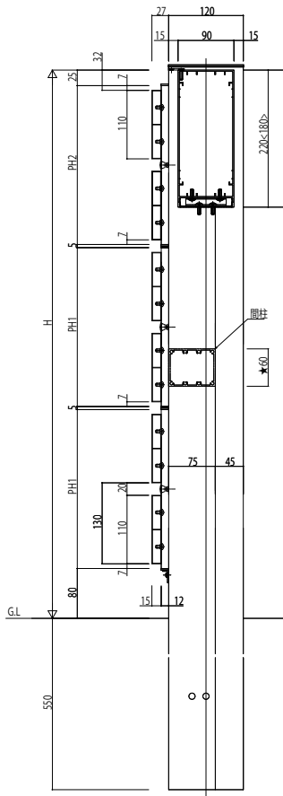
ウォールタイプ納まり図姿図
