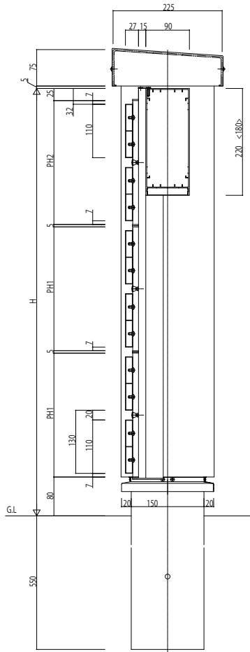
ウォールタイプ納まり図姿図
