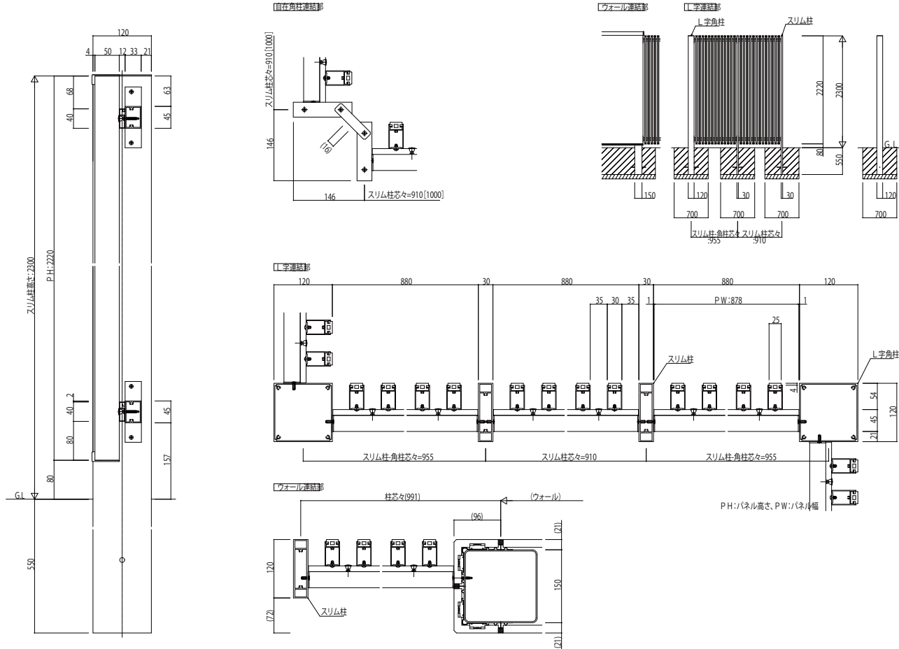
スリム自立式納まり図姿図
