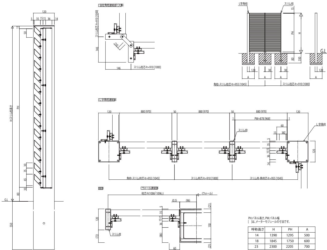
スリム自立式納まり図姿図
