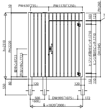
片開き姿図
