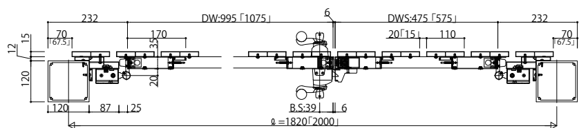
親子開き
