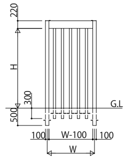
姿図(1:20)
