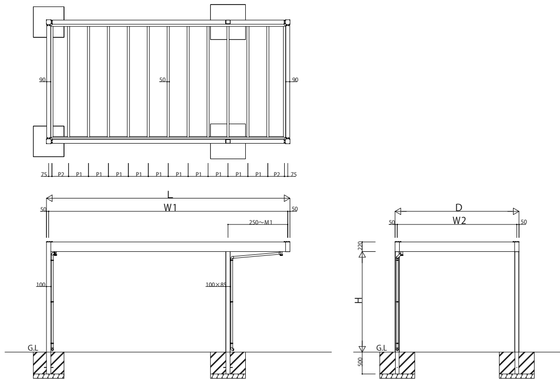
本図は【関東間 5427 H23】を表す。
