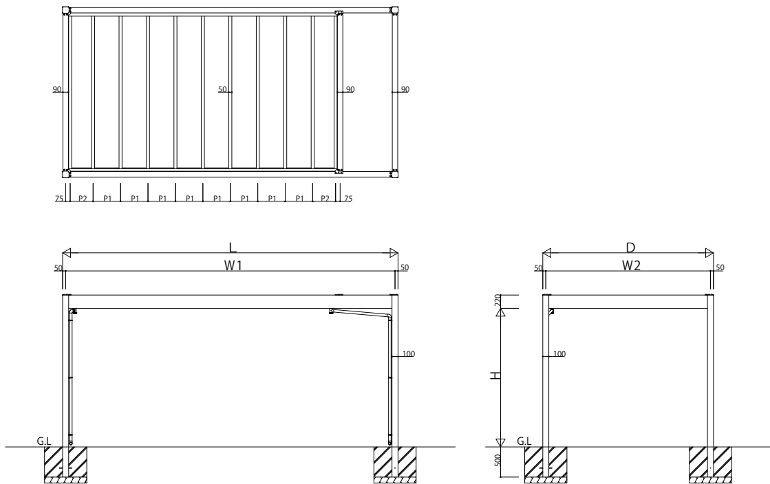
本図は【関東間 5427 H23】を表す。
