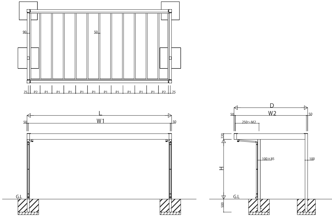
本図は【関東間 5427 H23】を表す。
