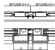
●4枚建突合せ部
