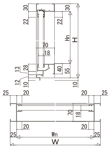
●ALC納まり 複層
