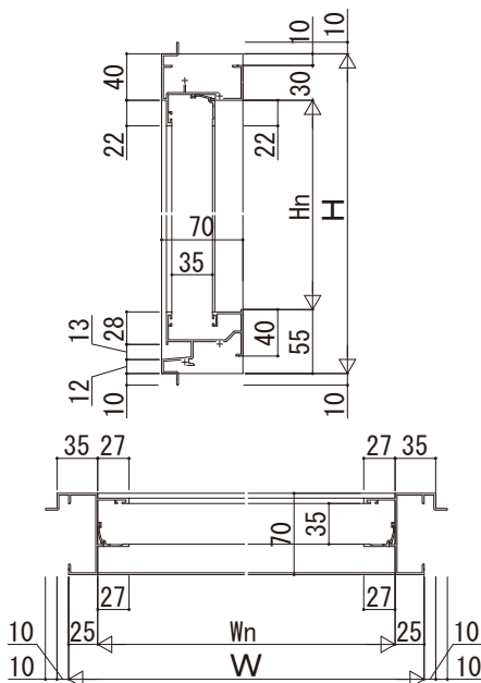
●ALC納まり 複層
