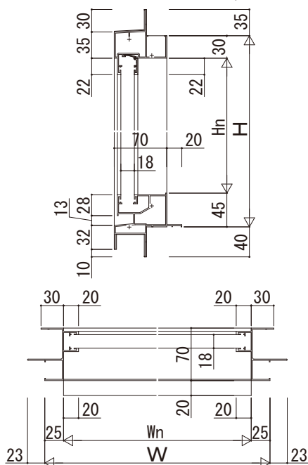
●RC納まり 複層
