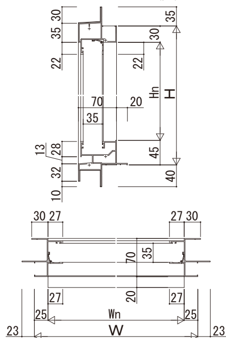
●ALC納まり 単板
