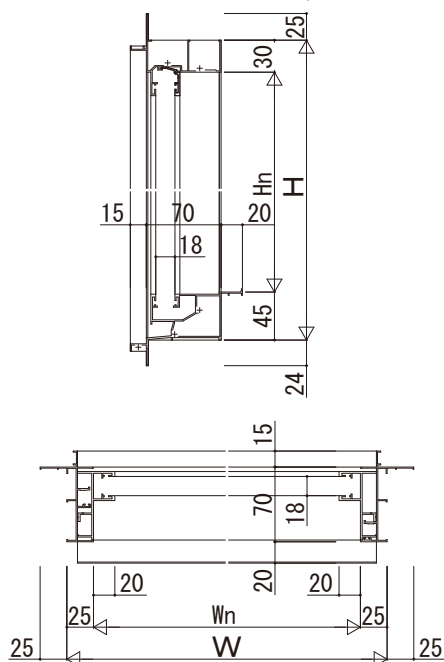
●RC納まり 単板
