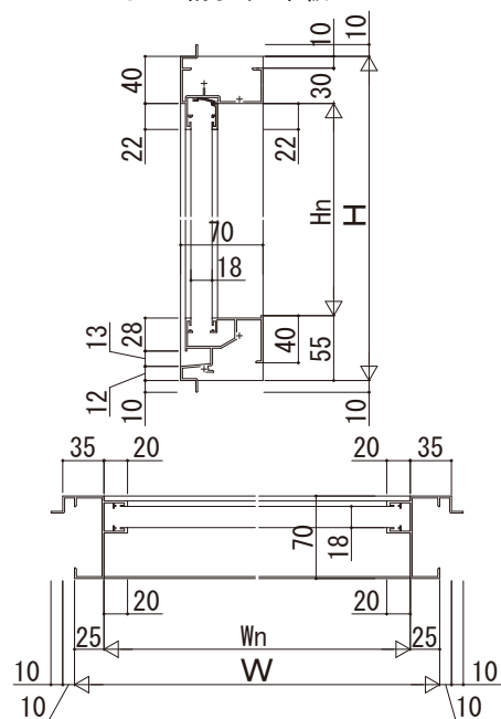
●ALC納まり 単板
