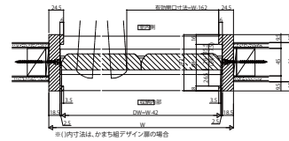
●横断面図 1枚折戸(3尺)
