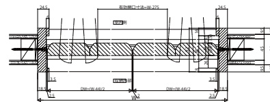
●横断面図 2枚折戸(4.5尺・6尺)
