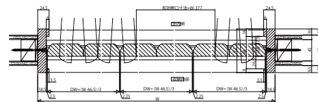
●横断面図 3枚折戸(9尺)
