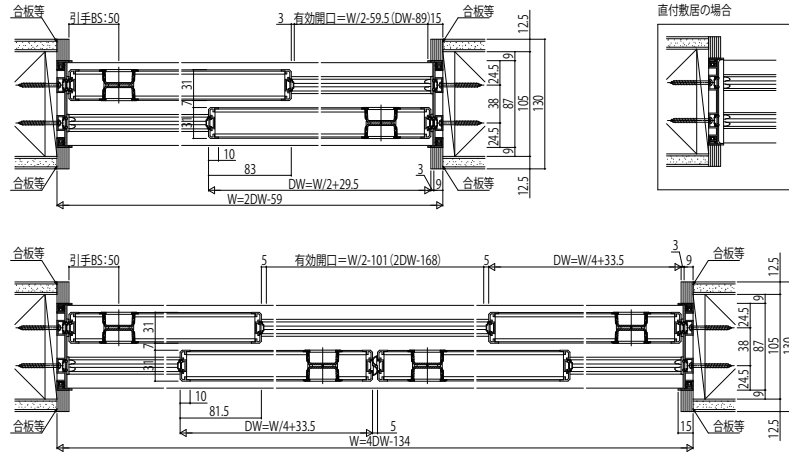
C11デザイン 採光部寸法 C11デザインはクローゼット引戸の設定なし。
