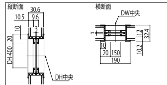
C11デザイン 採光部寸法 C11デザインはクローゼット引戸の設定なし。
