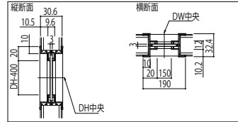
C11デザイン 採光部寸法 C11デザインはクローゼット引戸の設定なし。
