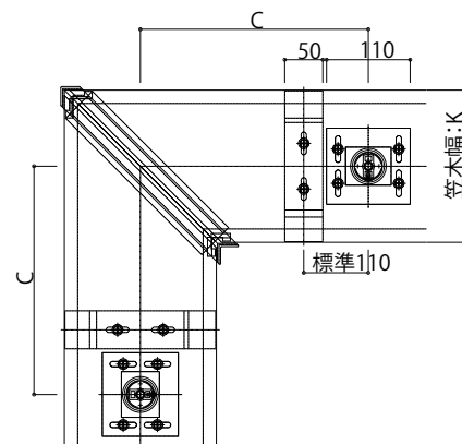
キャップ式コーナー 内勾配笠木
