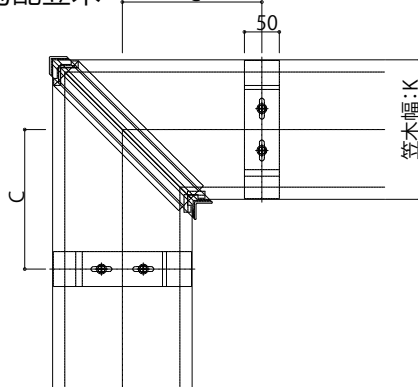
キャップ式コーナー 内勾配笠木
