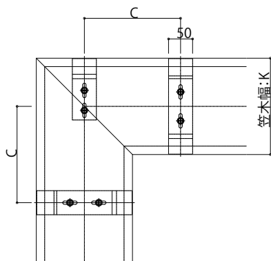
キャップ式コーナー 内勾配笠木
