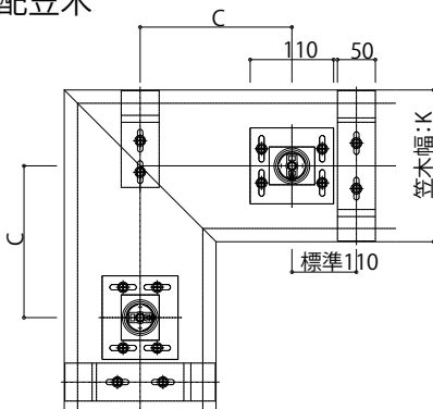
接着式コーナー 内勾配笠木
