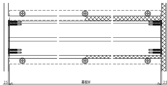
■正面図
